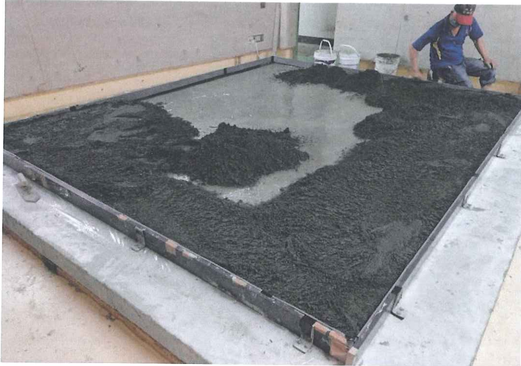
圖6.3 試件施工
